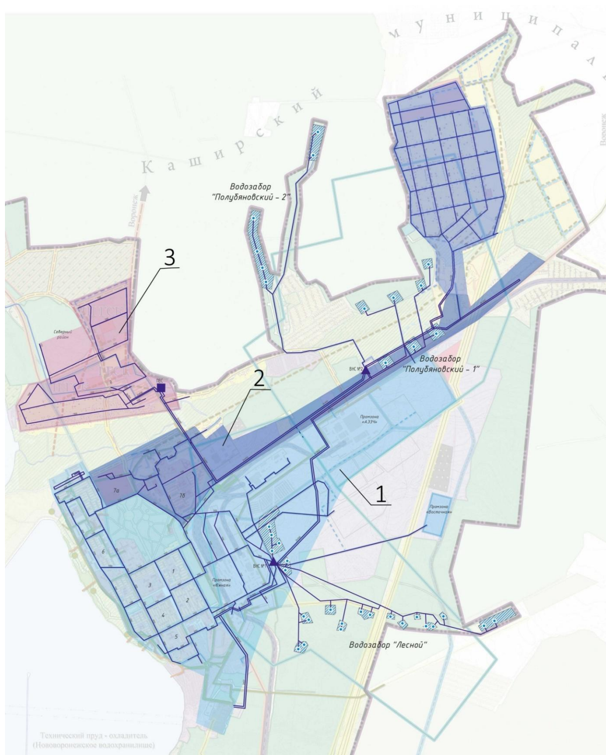
Технологические зоны централизованной системы водоснабжения 1 – технологическая зона ВНС № 1; 2 – технологическая зона ВНС № 2; 3 – технологическая зона ПВС.
