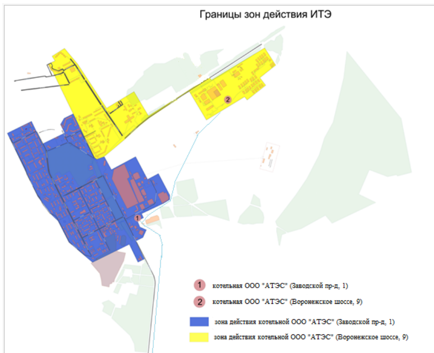
Рисунок 2.2.2. Зоны действия водогрейных котельных г. Нововоронежа
