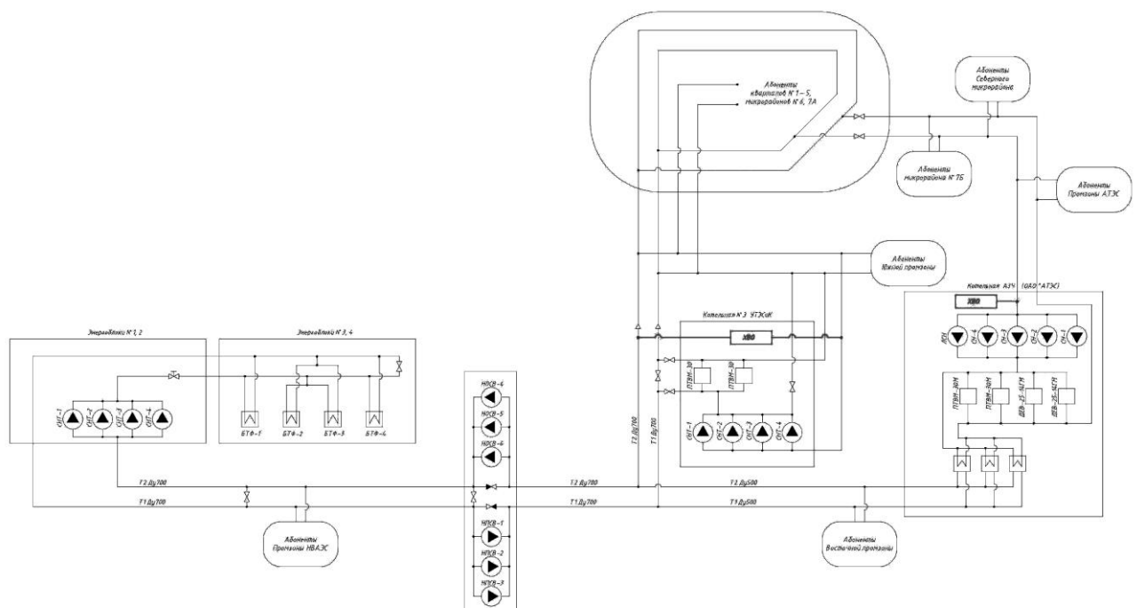
Рисунок 2.2.1. Структурная схема теплоснабжения г. Нововоронежа
