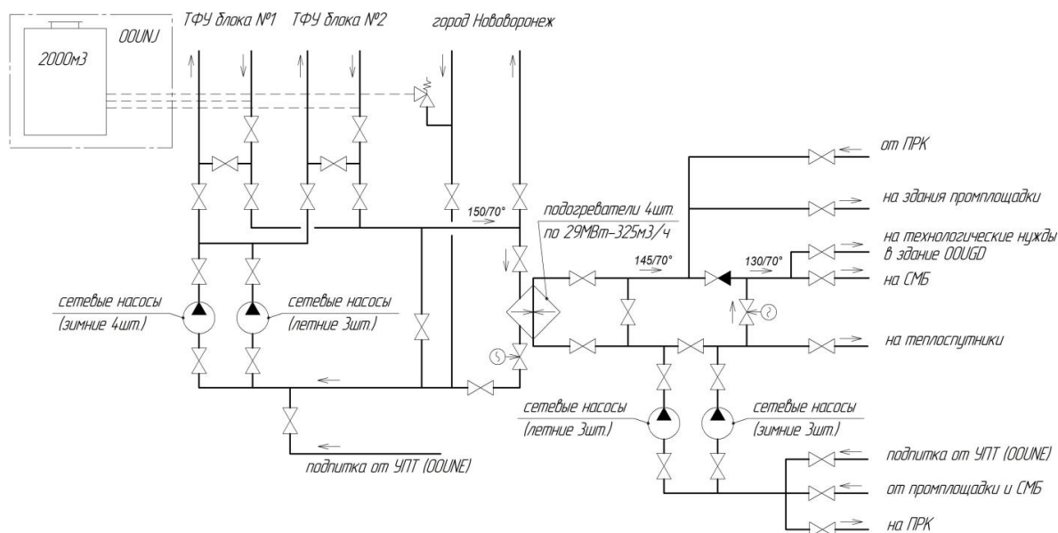
Схема включения теплораспределительного пункта в систему теплоснабжения
