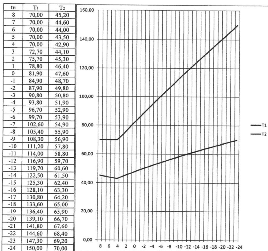
Температурный график
